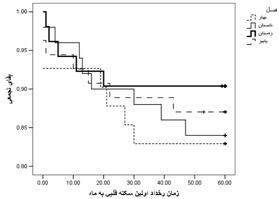
شکل ۱: منحنی تابع بقای تجمعی ۵ ساله بیماران سکنه قلبی حاد در بندر بوشهر بر حسب فصول سال و به تفکیک جنس طی سالهای ۸۰-۱۳۷۶
