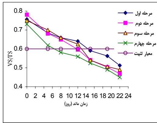
نمودار ۱: روند تغییرات نسبت VS/TS در چهار مرحله هضم
