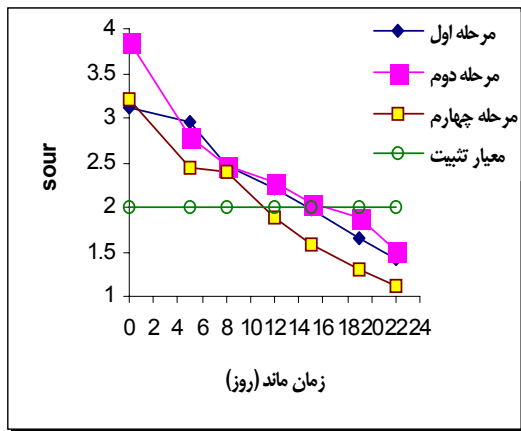
نمودار ۳: روند تغییرات Sour در مراحل اول، دوم و چهارم هضم
